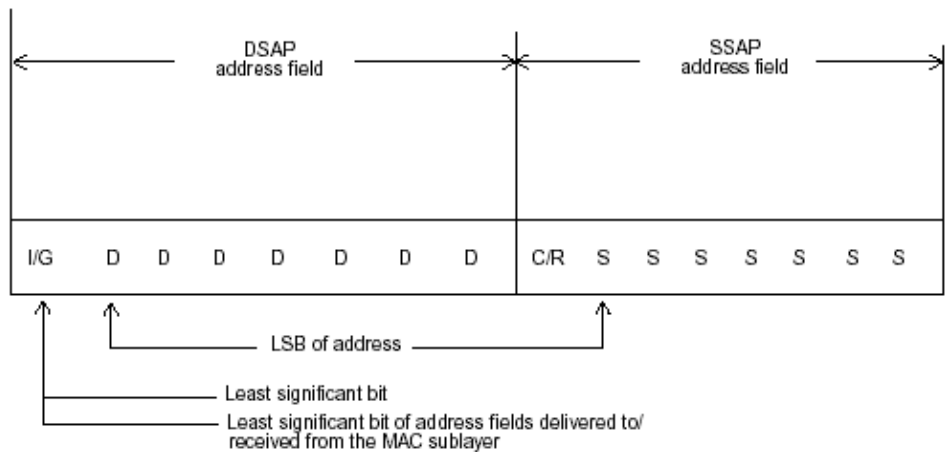
Fig. 3-2 SAP Format
