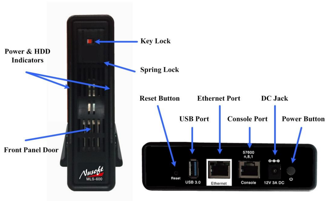
圖 H-1 MLS-600 接孔、指示燈說明
