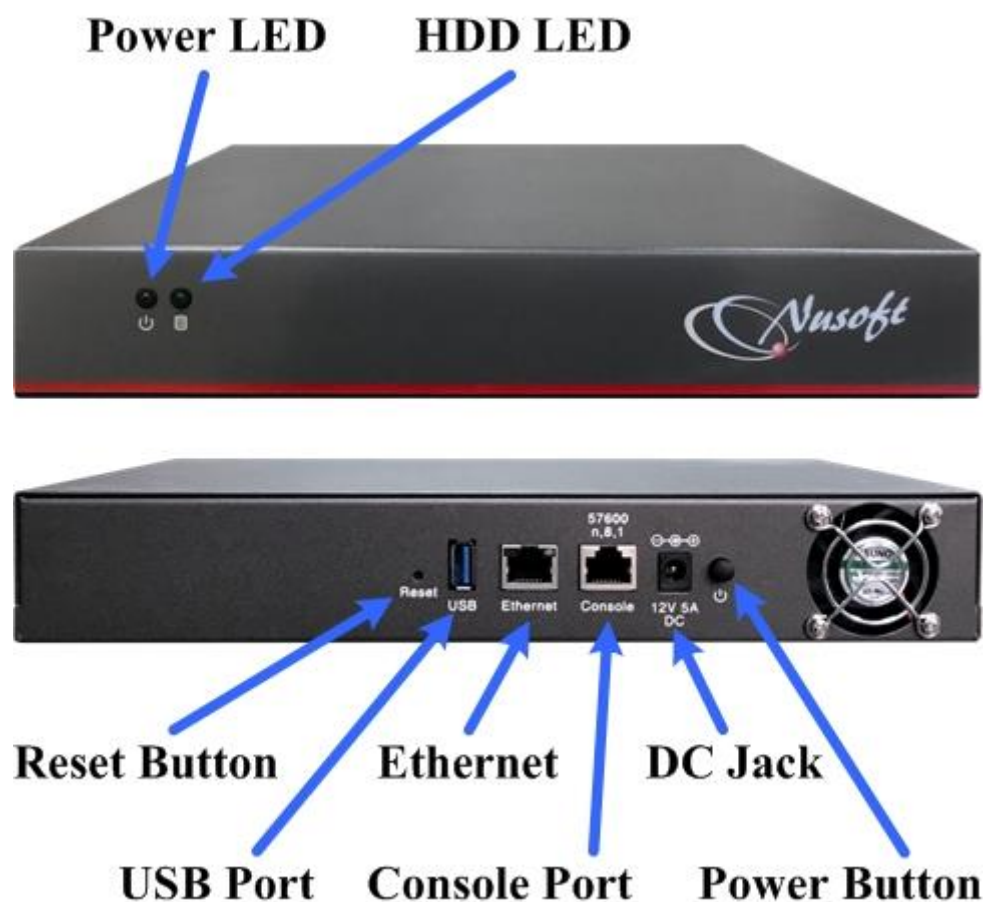
圖 H-2 MLS-600 接孔、指示燈說明
