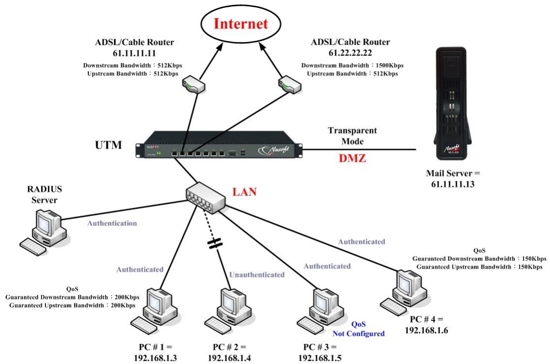
圖 H-8 MLS-600 配置圖
