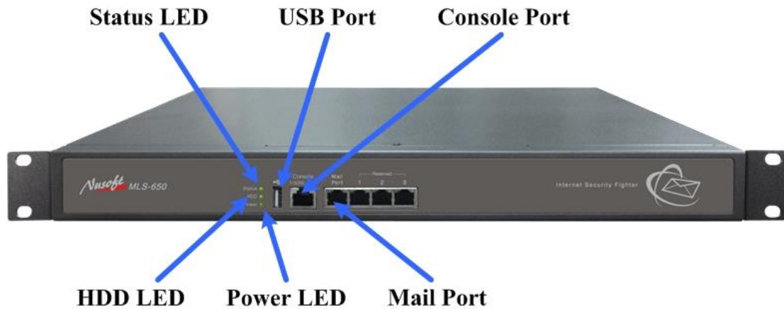
圖 H-1 MLS-650 接孔、指示燈說明
