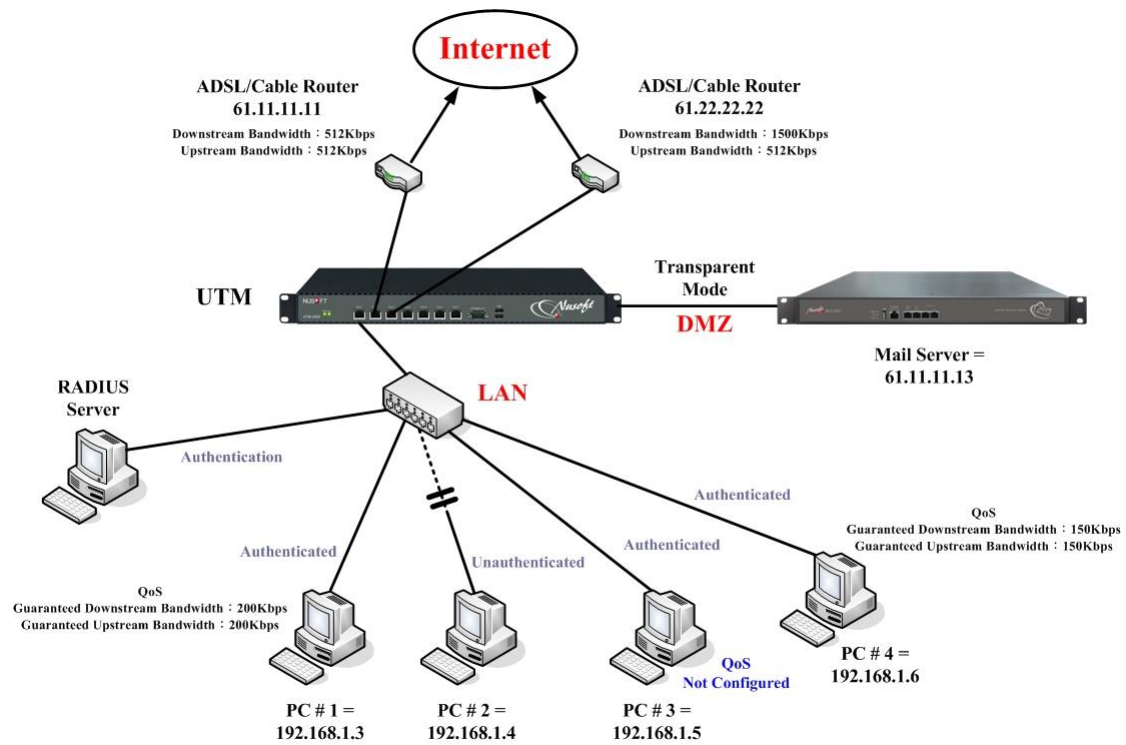
圖 H-2 MLS-650 配置圖
