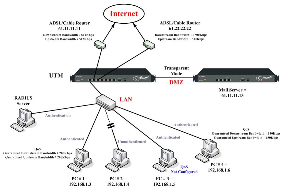
圖 H-2 MLS-1500C 配置圖
