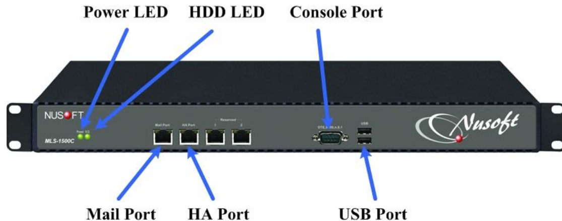
圖 H-1 MLS-1500C 接孔、指示燈說明
